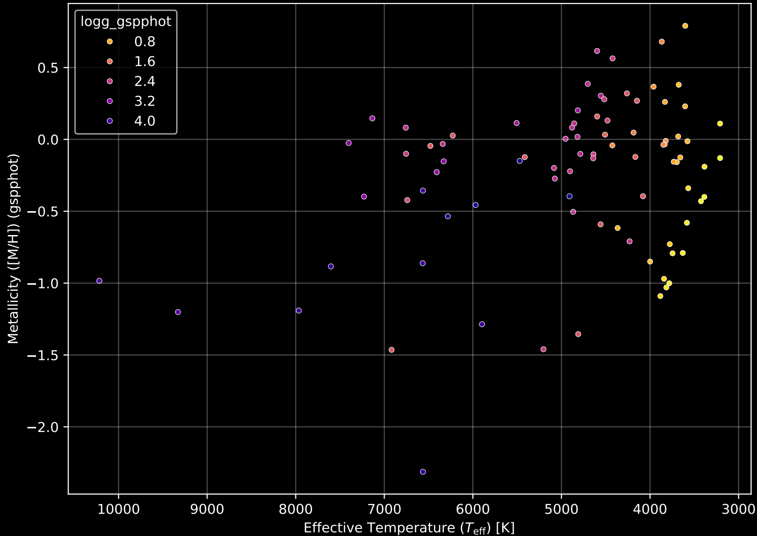
APOGEE DR17 Field: [002+04] Stellar Population Parameters (n= 86)
